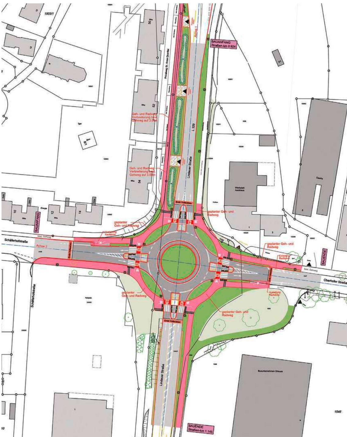
Kreisverkehr Oberhof-Schäferhof
